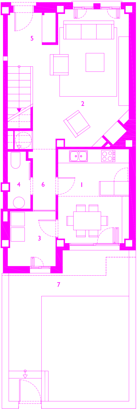
PLANTA BAJA/GROUND FLOOR
