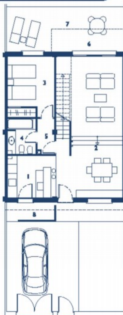
PLANTA BAJA/GROUND FLOOR
